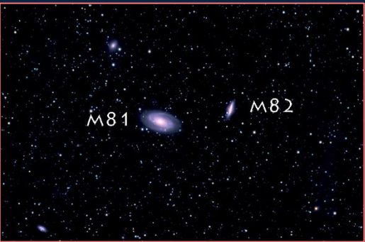
La galaxia del Cigarro (M82) en una imagen de campo amplio juntom a la galaxia de Bode (M81)
